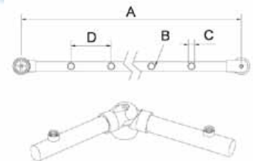
Dimensions/ Dimensiones
